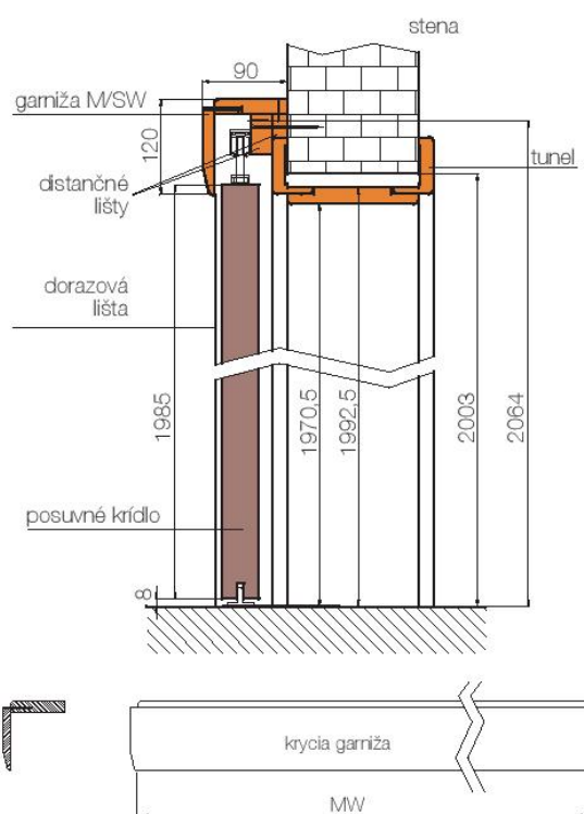
PŘÍKLAD POSUVNÉHO NASTENNÉHO SYSTÉMU S TUNELOM
