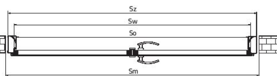
LIŠTA 60mm (L/MF) / 80mm (L/M8)
