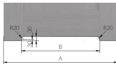
ventilačný výfrez (modely vyrábané v TECHNOLOGII RÁM SOFT)
