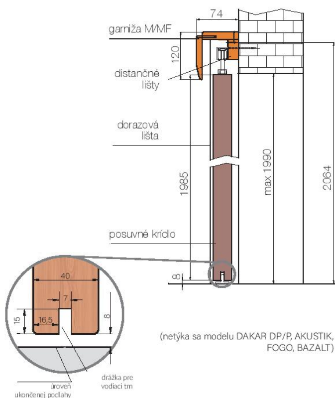
PŘÍKLAD POSUVNÉHO SYSTÉMU PŘÍMO NA STENU
