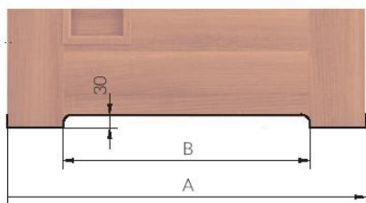
ventilačný výfrez (okrem modelov v TECHNOLOGII RÁM SOFT)
